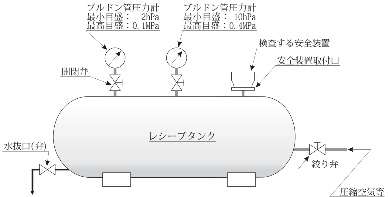
例 2 最高試験圧力 0.4 MPa の試験装置
