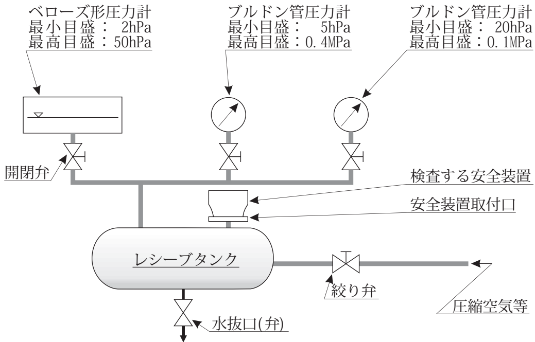
例 1 最高試験圧力 1 MPa の試験装置
